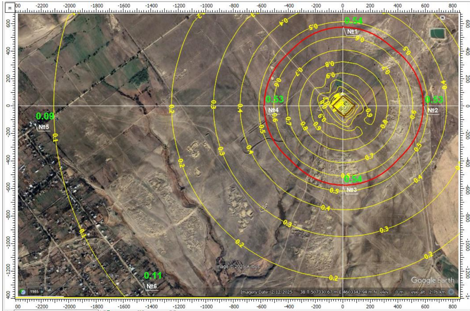
აზოტის დიოქსიდის (კოდი 301) მაქსიმალური კონცენტრაციები საკონტროლო წერტილებში (№№ 1-4 ნორმირებულ 500 მ-ს ზონის საზღვარზე, №№ 5 და 6 -უახლოეს დასახლებებთან
