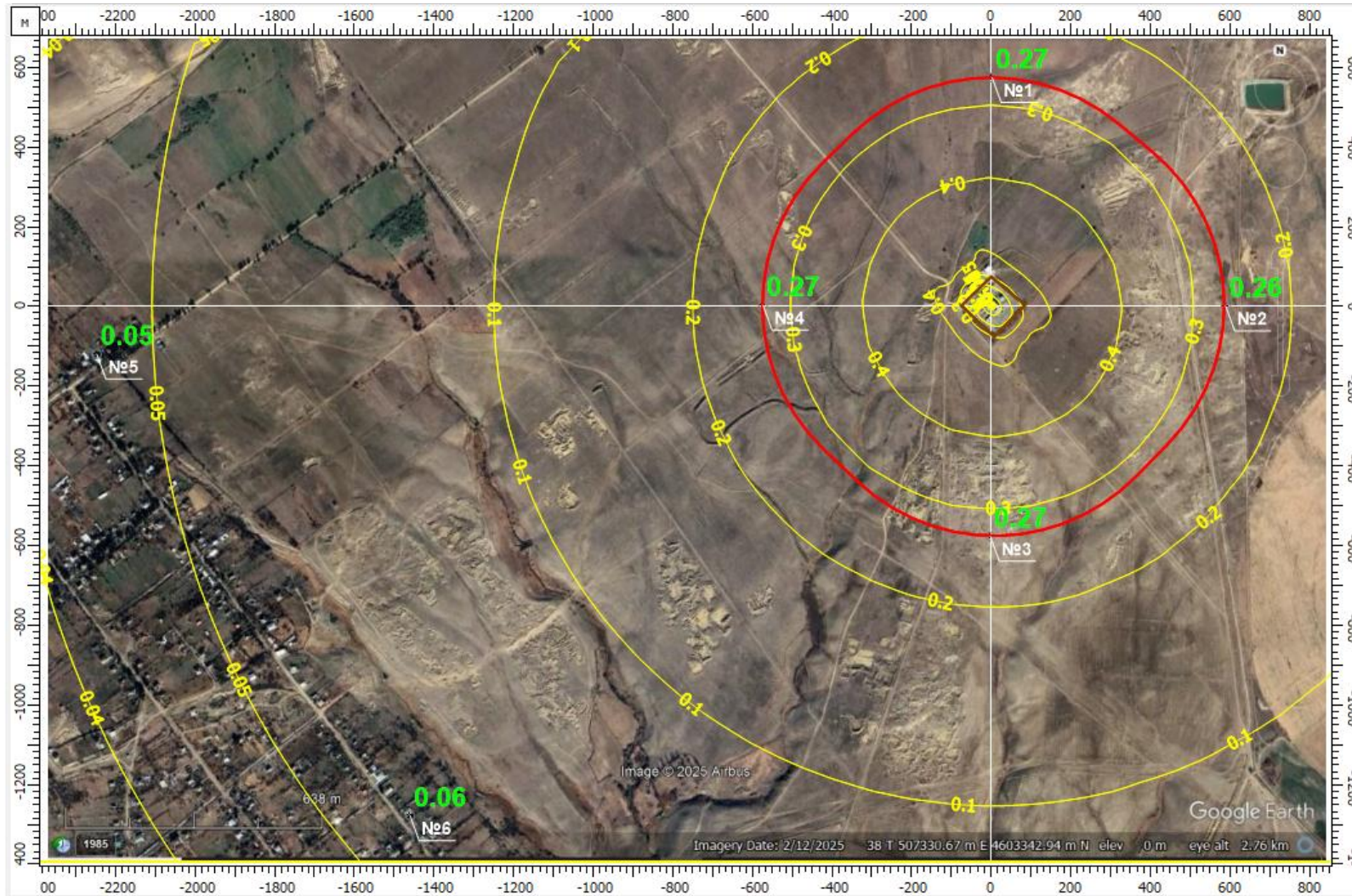
აზოტის ოქსიდის (კოდი 304) მაქსიმალური კონცენტრაციები საკონტროლო წერტილებში (№№ 1-4 ნორმირებულ 500 მ-ნ ზონის საზღვარზე, №№ 5 და 6 -უახლოეს დასახლებებთან
